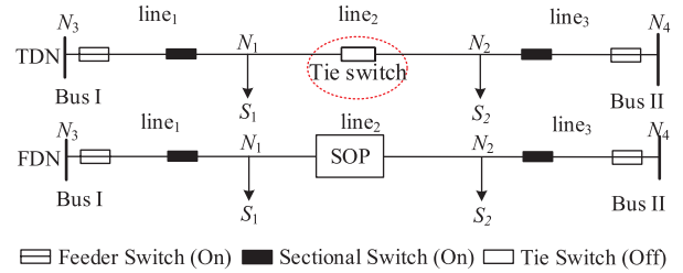
Fig. 5. Single-loop network case (overhead lines).
